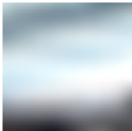
Bicubic 18.9522 dB
