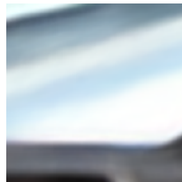
SC-INR+PhiZ 23.1429 dB
