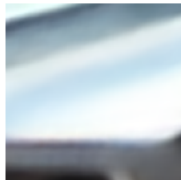
SC-INR 21.6285 dB
