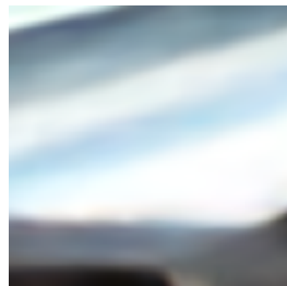
LTE 21.2079 dB
