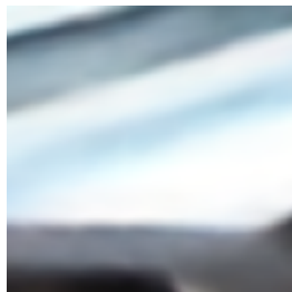
LIIF 20.1493 dB
