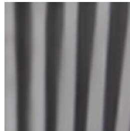
SC-INR+PhiZ 13.3548 dB
