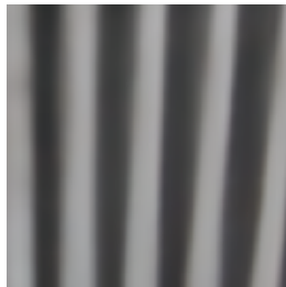
LTE 13.4507 dB
