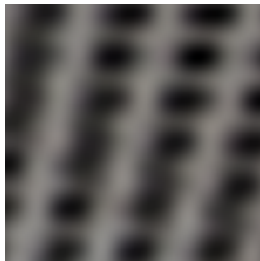
Bicubic 16.2966 dB
