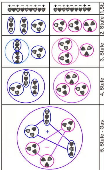
Der Aufbau von Wasserstoff, Variante 9+ 9-
