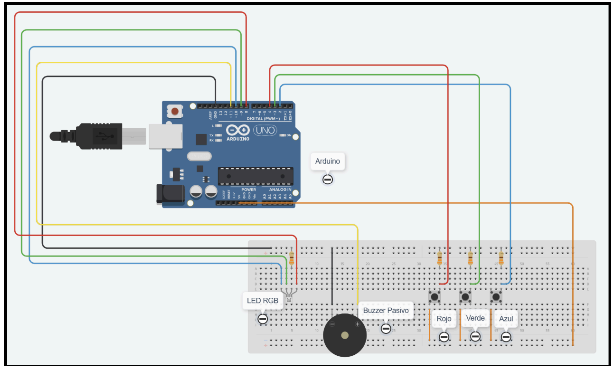
Figura 1: Diagrama de las conexiones del sistema utilizado, incluyendo descripciones de los componentes principales del circuito electrónico (no se utilizó el Arduino Mega utilizado en el circuito verdadero dado a que no había un modelo disponible). [Diagrama hecho con Tinkercad]
