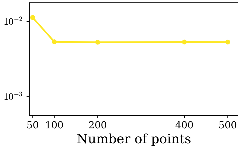
Lotka-Volterra
