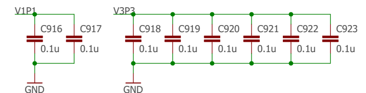
MCU Decoupling
