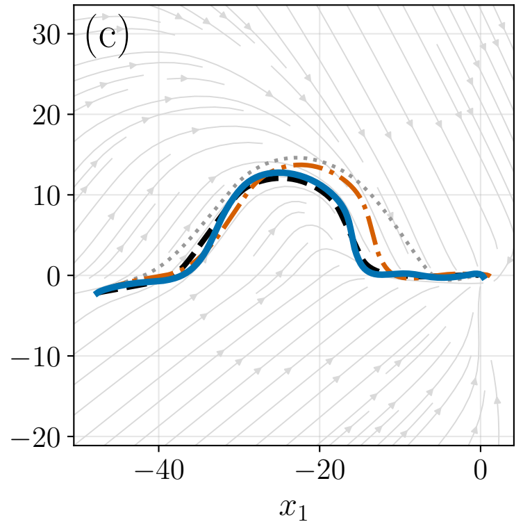
LASA: Worm
