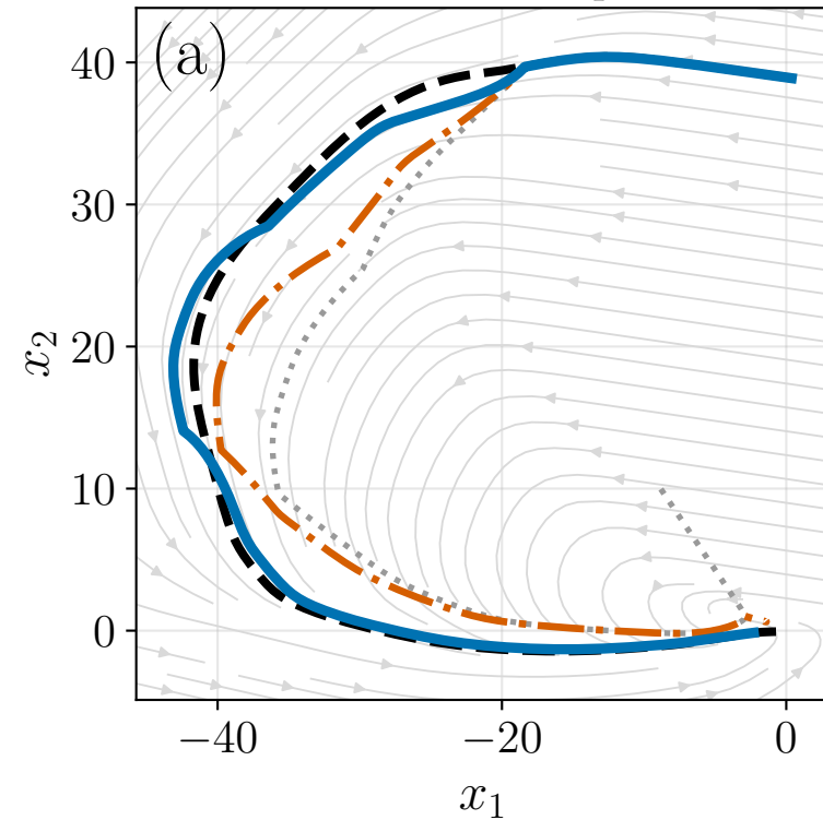
LASA: CShape
