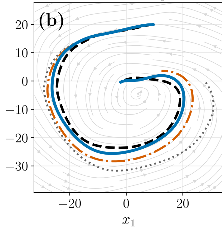
LASA: GShape
