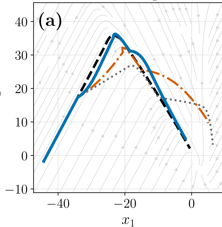
LASA: Angle
