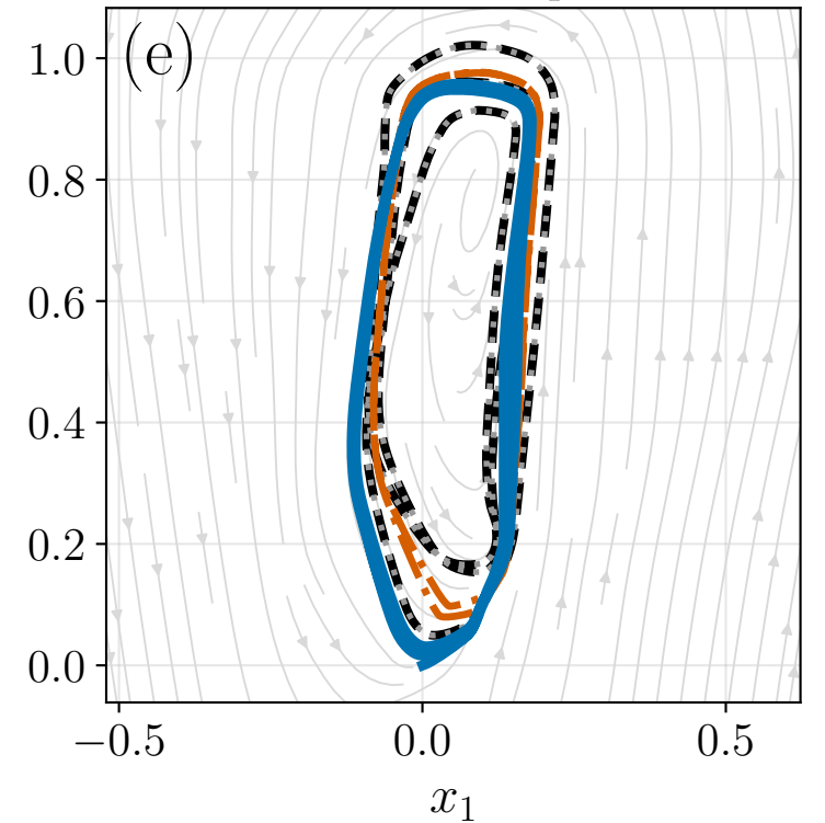
IROS: IShape
