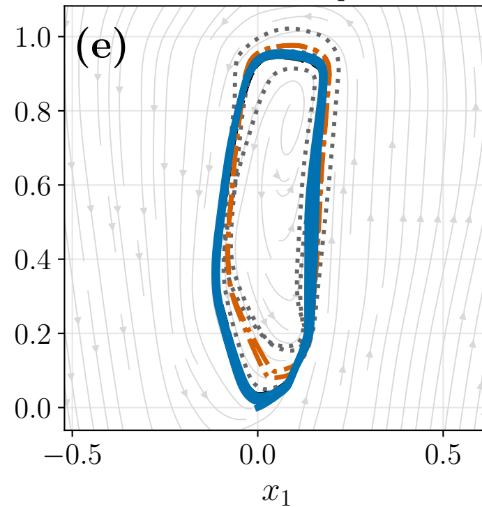
IROS: IShape
