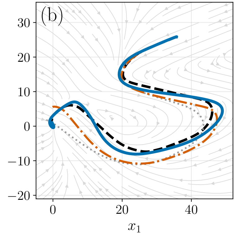
LASA: Snake
