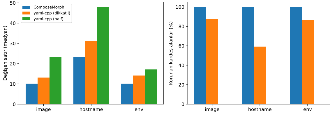
Şekil 1. ComposeMorph ile iki ham yamll-cpp kullanımının karşılaştırması (Veri Kümesi B). Solda düzenleme başına değişen satır sayısının medyanı, sağda düzenlenen servisin diğer alanlarının korunma oranı. Alt ağacı yeniden inşa eden saf kullanım hiçbir vakada kardeş alanları koruyamamaktadır (%0, çubuk görünmez). Dikkatli kullandaki eksik, tırnak kaybı sonucu tip değişiminden kaynaklanır; kardeş alanlar yapısal olarak yerindedir.
