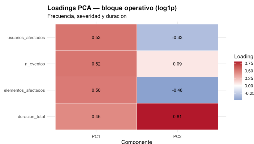
Figura 5.45: Peso (loadings) de frecuencia, afectación y duración en las dos primeras componentes del bloque operativo.
