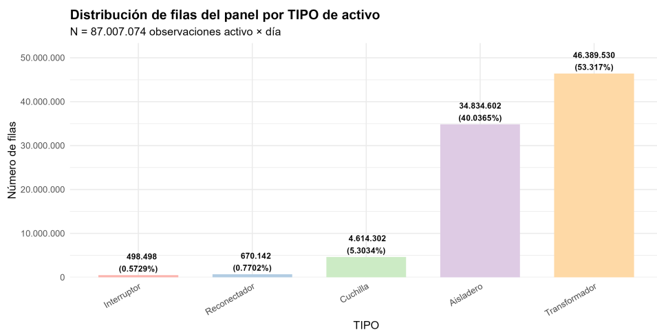
Figura 5.12: Distribución de filas del panel por TIPO de activo ( N = 87,007,074 ).
