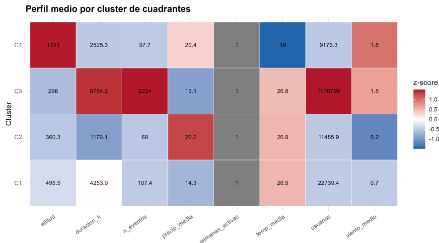
Figura 5.63: Perfil medio por cluster de cuadrantes (variables operativas y climáticas).
