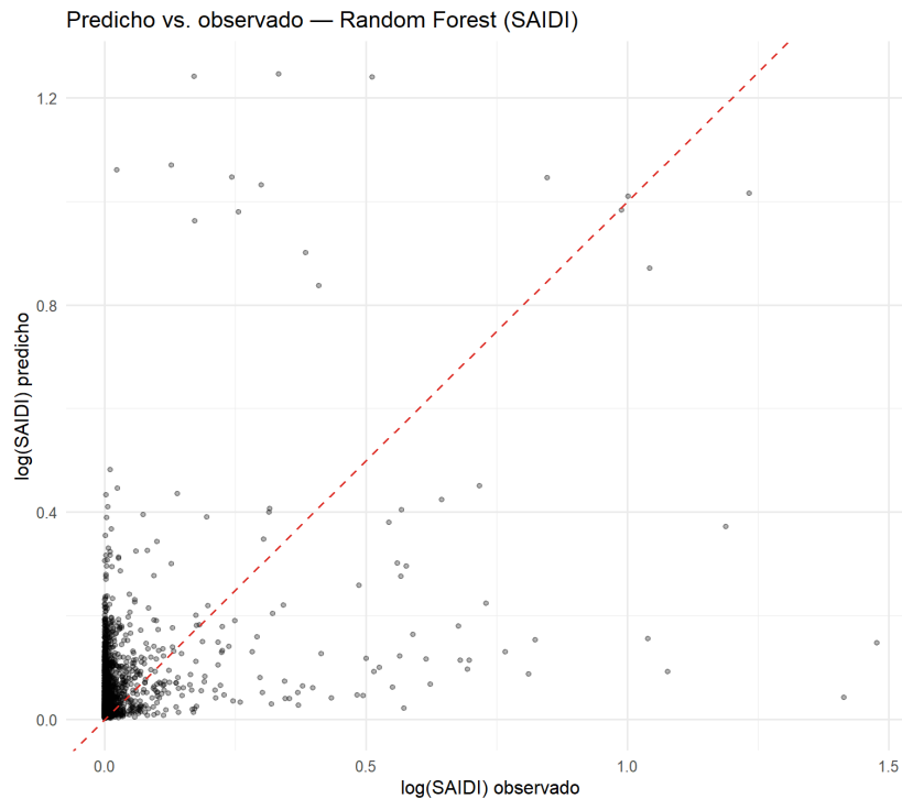
Figura 5.69: Valores observados frente a predichos de SAIDI en el conjunto de prueba (escala \log(1 + y) ).
