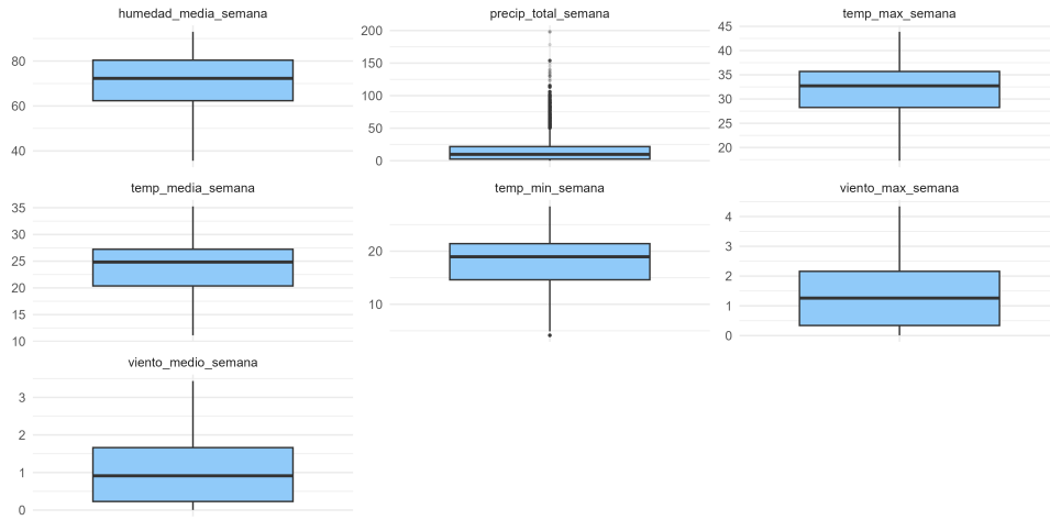
Figura 5.20: Distribución de las variables climáticas semanales: mediana y extremos ( N_{\text{agr}} = 90.128 ).
