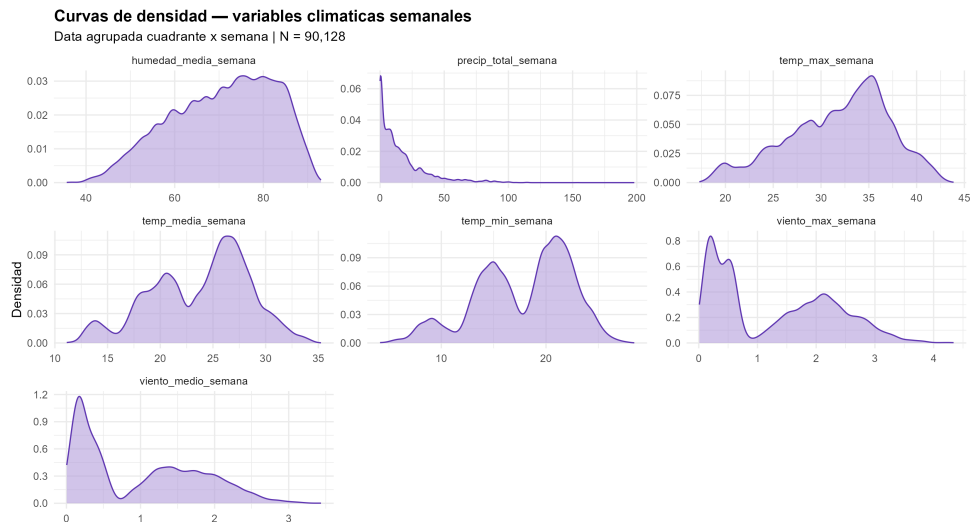
Figura 5.26: Forma de la distribución de las variables climáticas semanales ( N_{\text{agr}} = 90.128 ).
