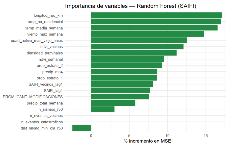
Figura 5.72: Importancia de variables (%IncMSE) del Random Forest para SAIFI .
