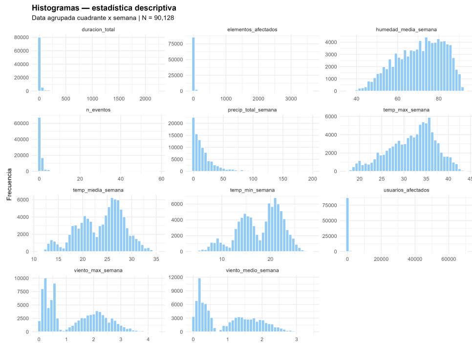
Figura 5.24: Distribución de las variables numéricas de la tabla agrupada: forma y cola ( N_{\text{agr}} = 90.128 ).
