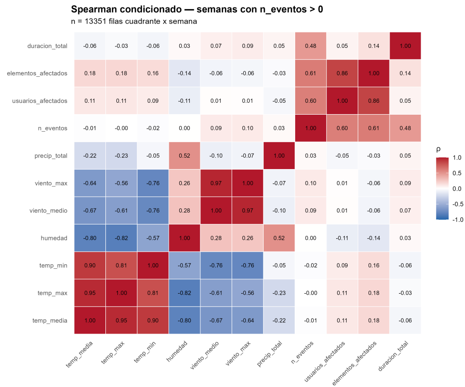
Figura 5.51: Correlaciones de Spearman en semanas-cuadrante con n\_eventos > 0 ( n = 13.351 ).
