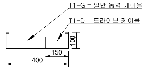
하단 트레이 단면도
