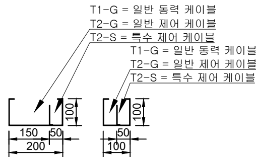
일반 덕트 단면도
