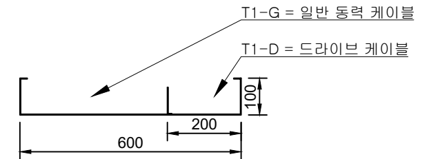
CR룸 하단 트레이 단면도
