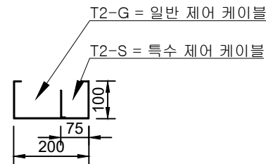
상단 트레이 단면도
