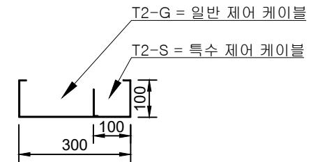
CR룸 상단 트레이 단면도
