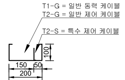
211/212/221/222/223 트레이 단면도
