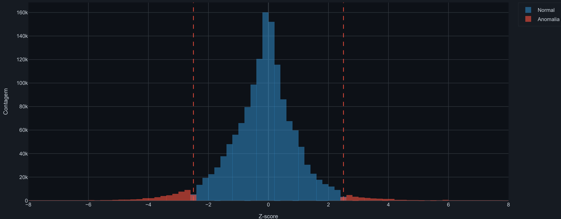
Distribuição de Z-scores
