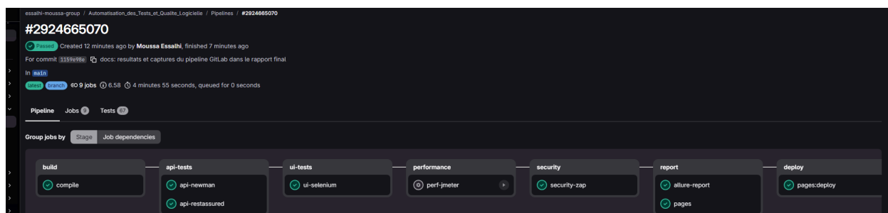
Figure 6 - Pipeline GitLab réussi : graphe réel des stages (capture du pipeline #2924665070)
