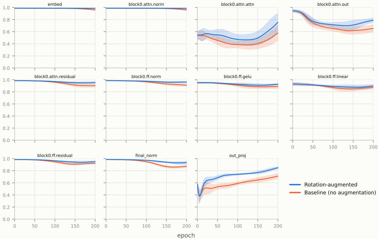
linear CKA
