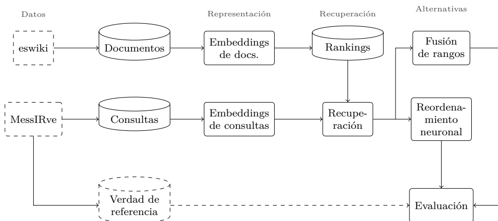
Figura 4.1: Arquitectura del sistema de recuperación. Los documentos provienen del corpus de la Wikipedia en español (eswiki) y las consultas y los documentos relevantes, del conjunto de datos MessIRve. La fusión de rangos y el reordenamiento neuronal se evalúan como alternativas sobre la misma lista de candidatos, no como etapas sucesivas.
