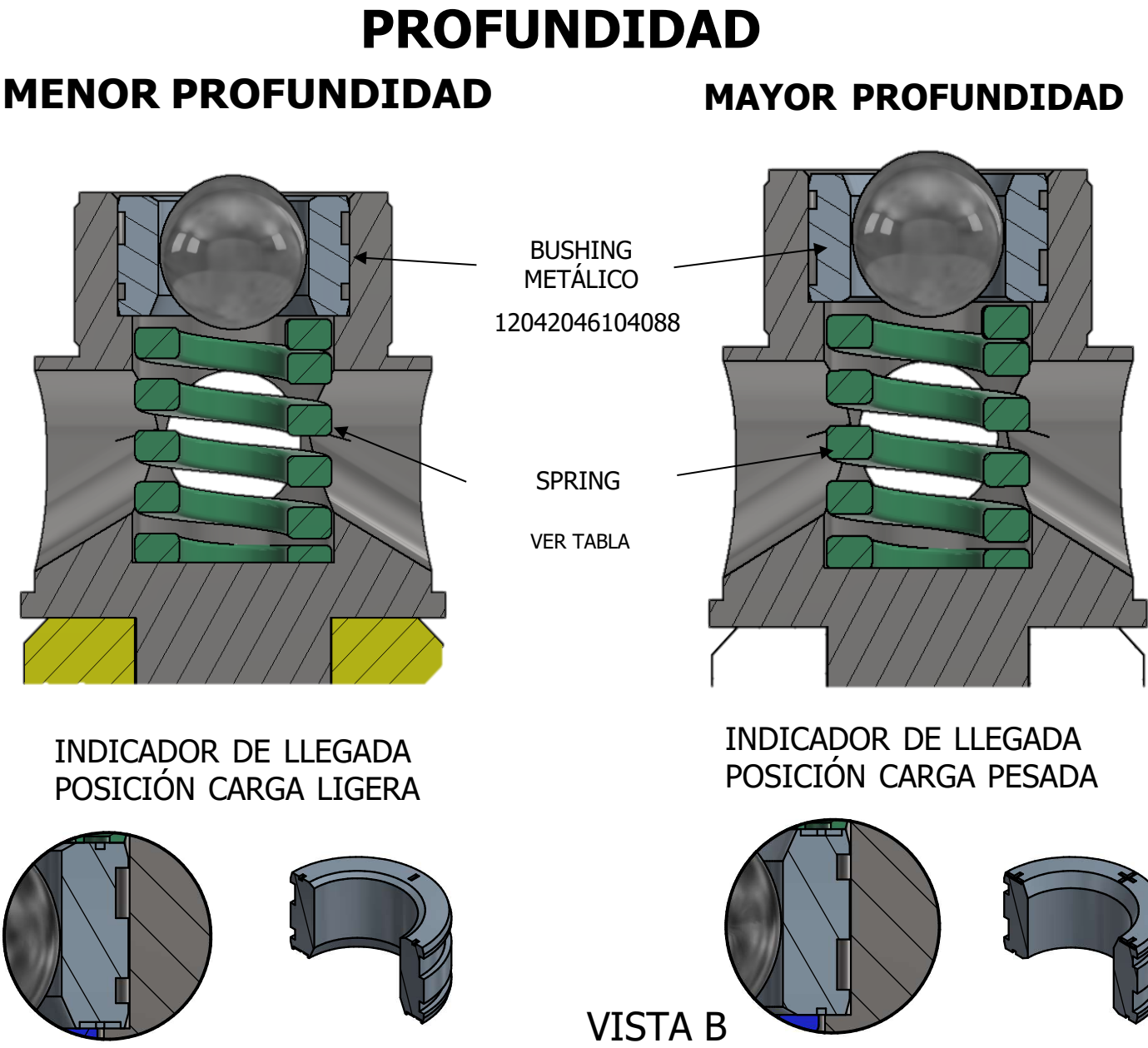
KIT DE RETENCIÓN POZO SECO
