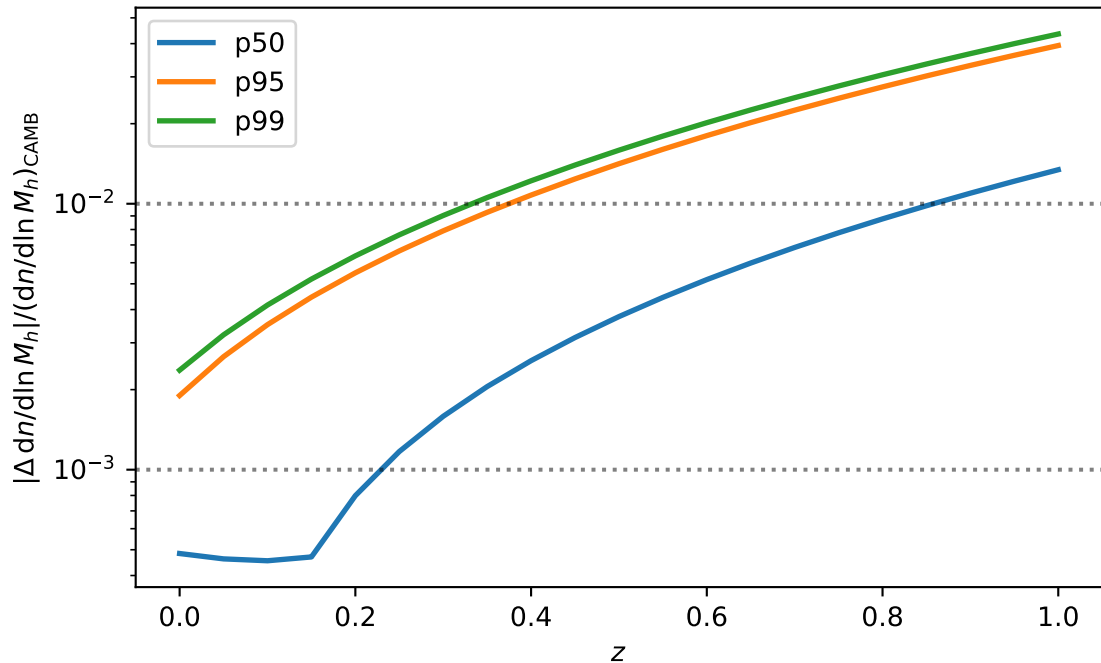
HMF error vs. z (cluster mass band 10^{13} -- 10^{15} M_{\odot}/h )
