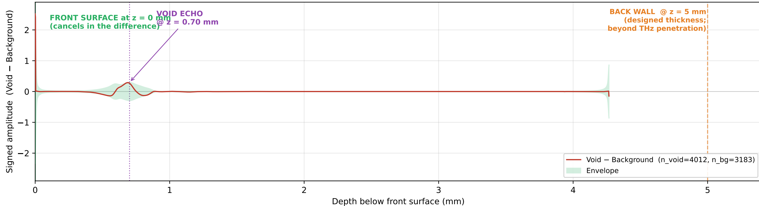
Sample 4 · CV04 · 4 cylindrical voids
