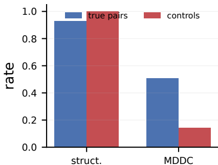
(d) BigVul tradeoff
