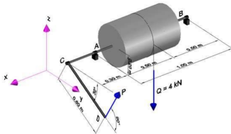
Figura 4: Cilindro con polea y contrapeso — Ejercicio 4.
