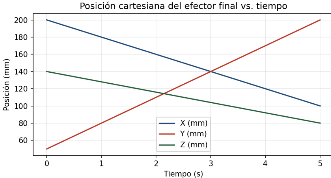
Figura 2. Posición cartesiana X, Y, Z del efector final en función del tiempo.
