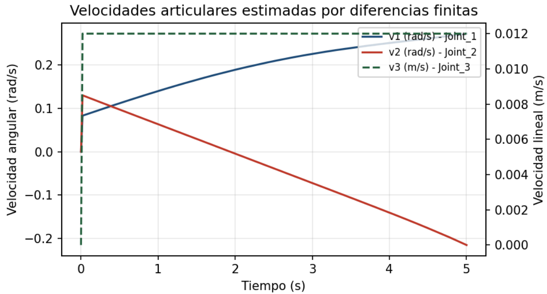
Figura 3. Velocidades articulares v_1 , v_2 (rad/s) y v_3 (m/s) estimadas por diferencias finitas.
