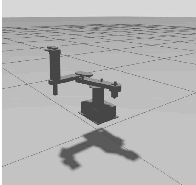
Figura 1. Posición final del efector final del robot SCARA R4 en Gazebo Sim ( t = 5.00 s, P1 = (100, 200, 80) mm).
