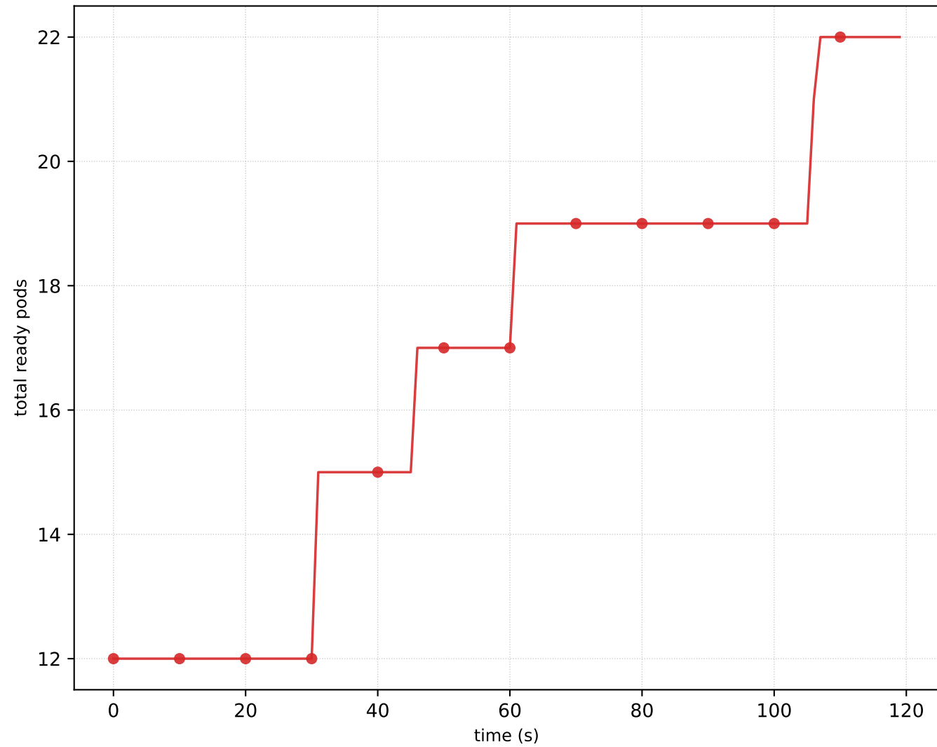
istio
