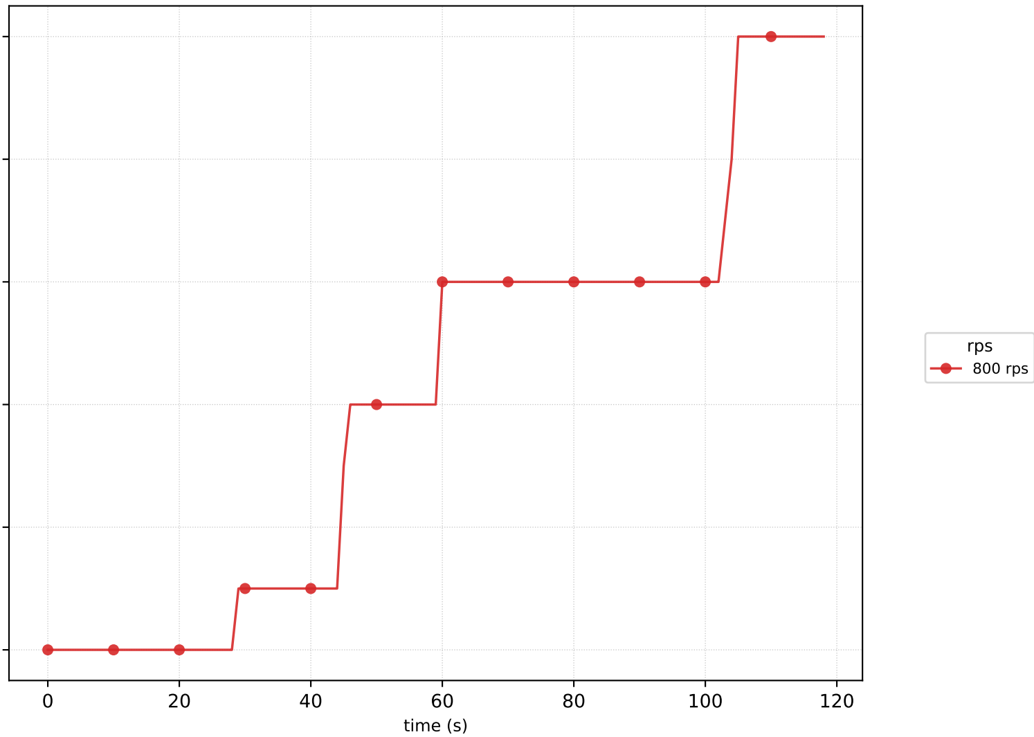
st5-AttUpd
