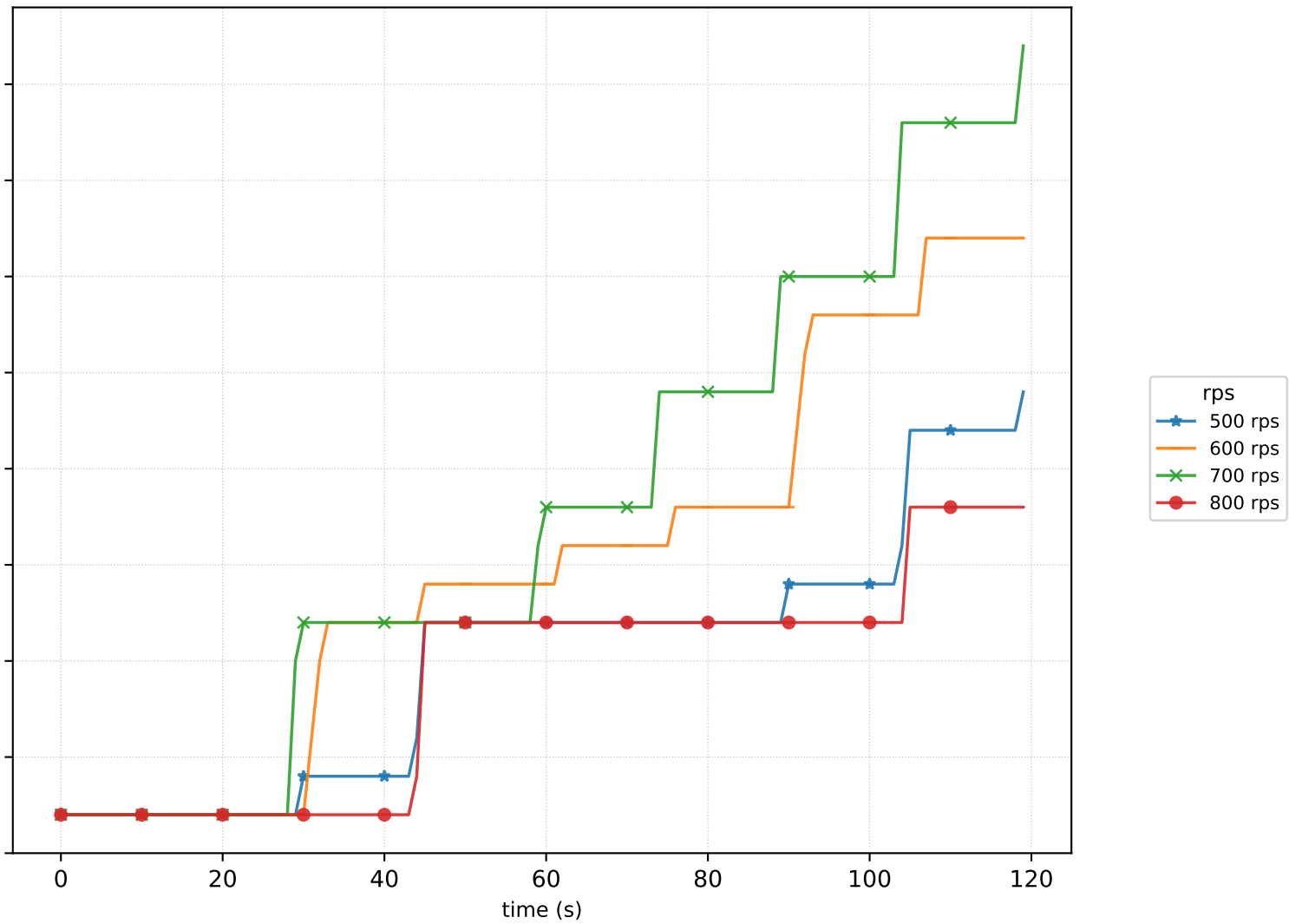
st5-AttUpd
