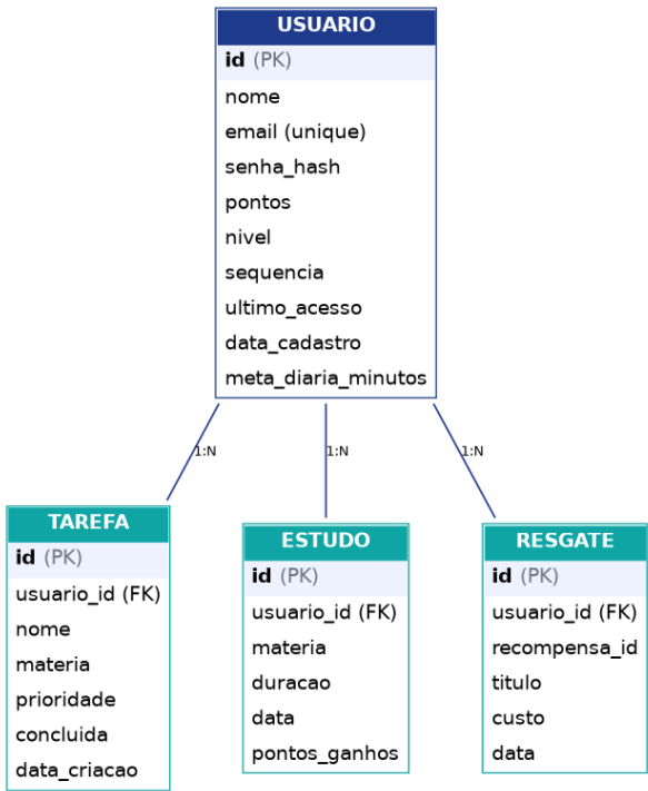
Figura 1: Modelo de dados do protótipo (diagrama entidade-relacionamento).
