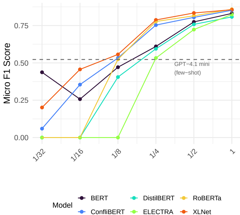
a. F1 vs. Training Data Fraction
