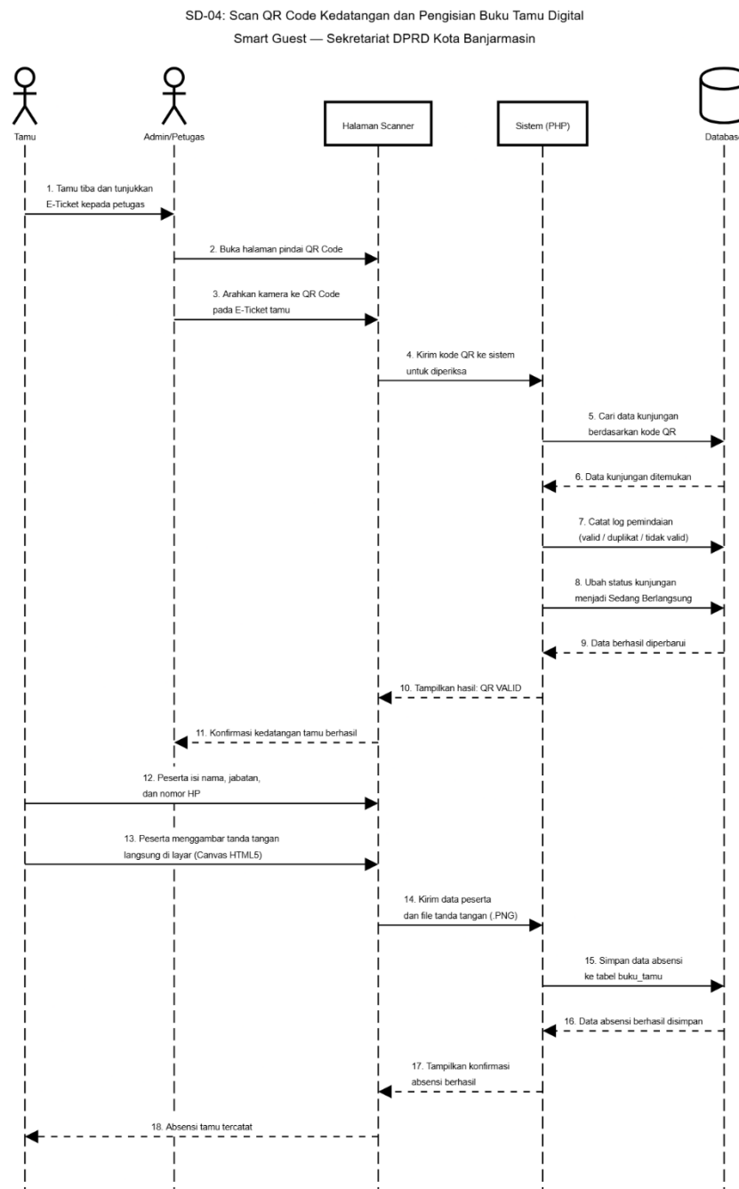
Gambar 3. 6 Sequence Diagram Scan QR Code dan Pengisian Buku Tamu
