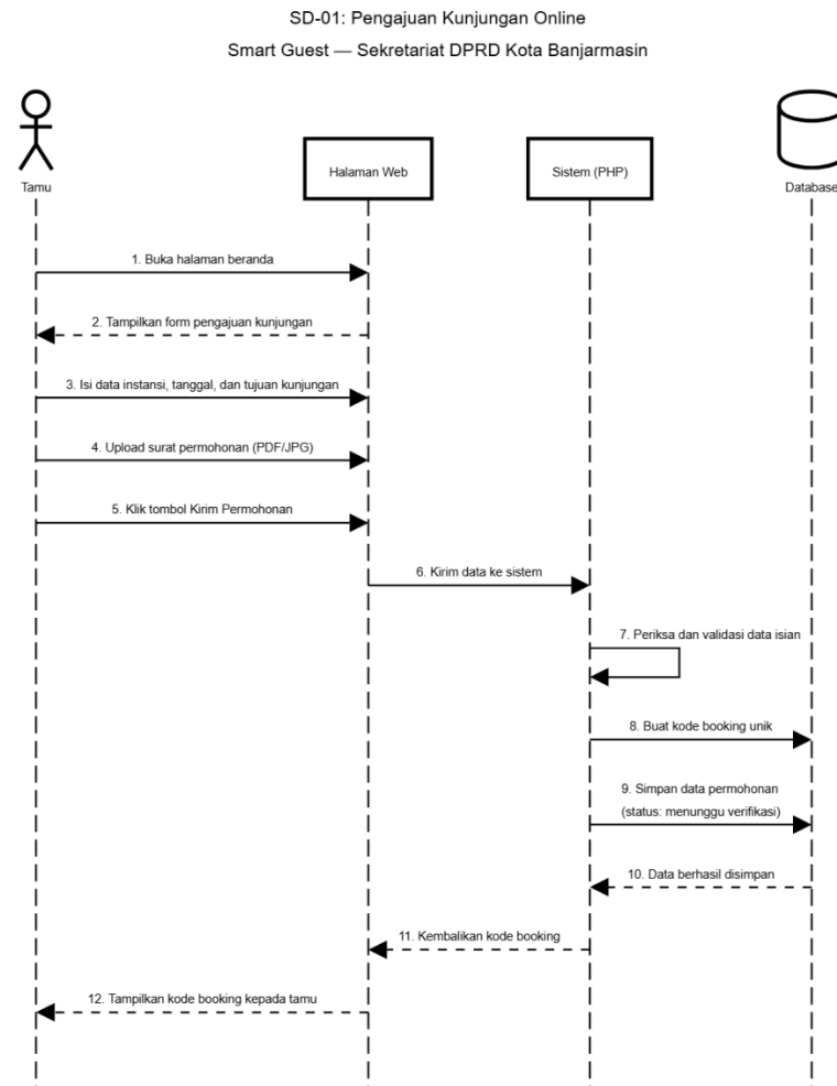
Gambar 3. 3 Sequence Diagram Pengajuan Kunjungan Online
