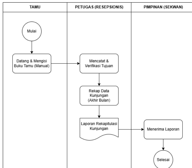
Gambar 3. 1 Flowmap Sistem yang Berjalan
