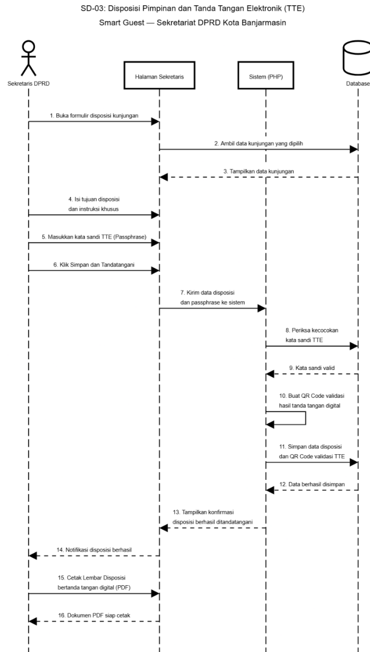
Gambar 3. 5 Sequence Diagram Disposisi Pimpinan dan TTE
