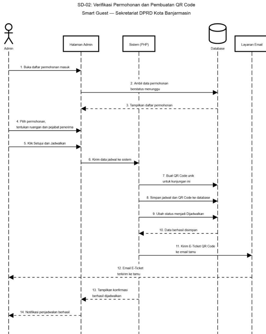
Gambar 3. 4 Sequence Diagram Verifikasi Permohonan dan Pembuatan QR Code
