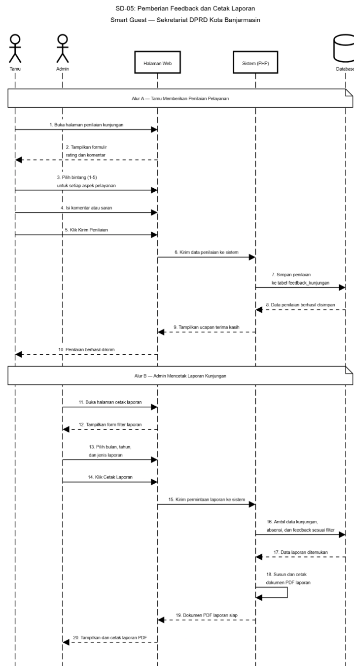
Gambar 3. 7 Sequence Diagram Pemberian Feedback dan Cetak Laporan
