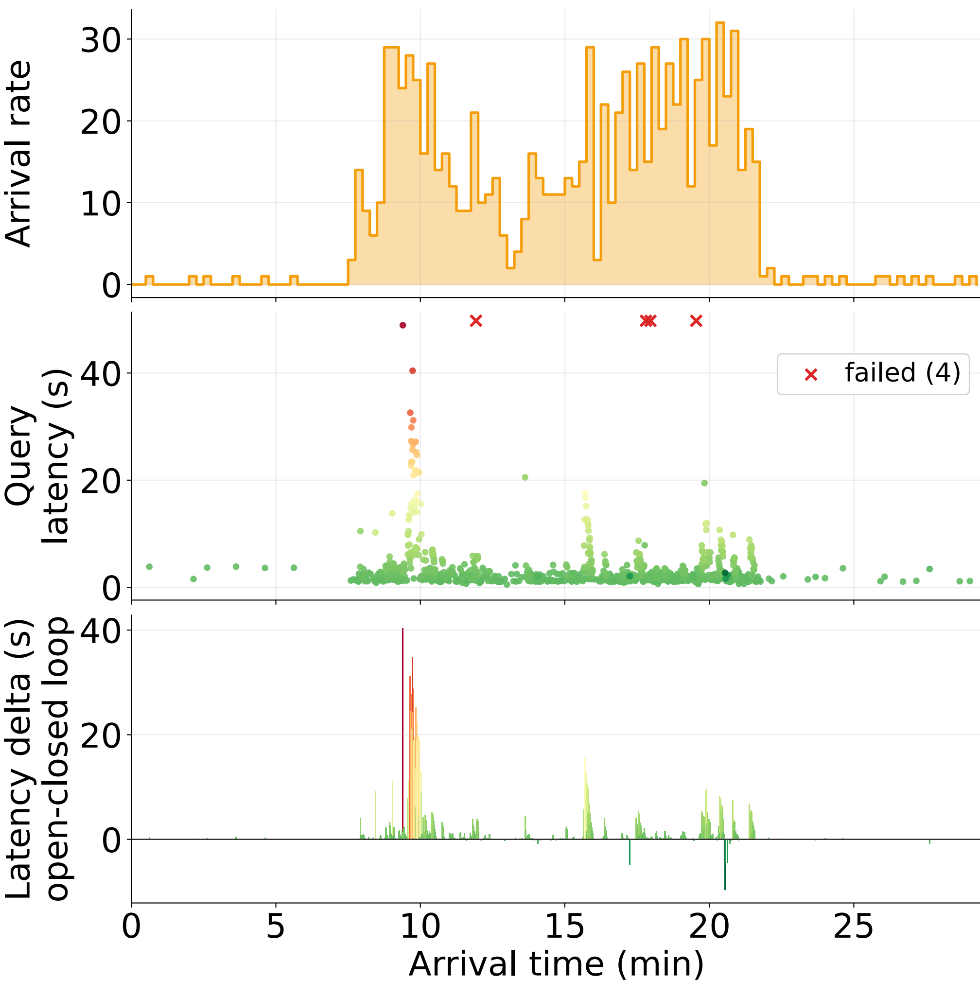
Trino
