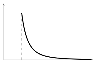
D.13 Pareto (Power Law)
