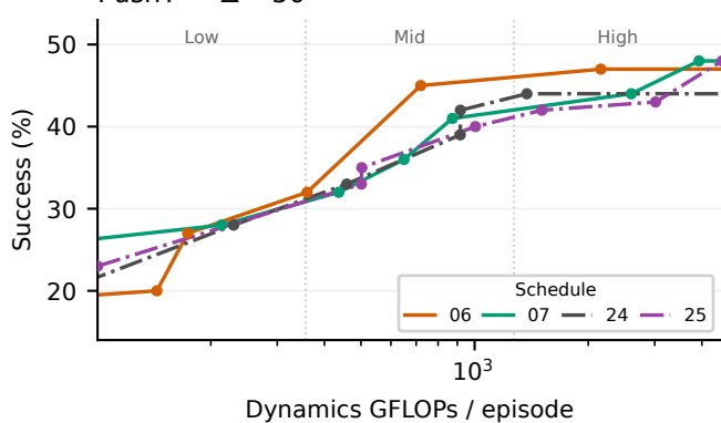
PushT — \Delta = 50
