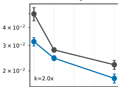
NPO / forget05
