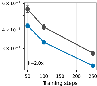
SimNPO / forget05
