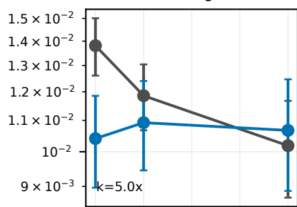
NPO / forget01
