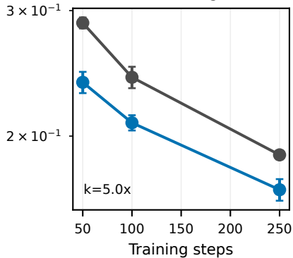
SimNPO / forget01
