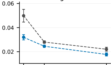
forget05
