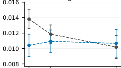
forget01
