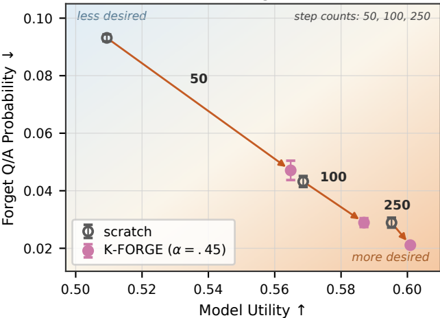
NPO
