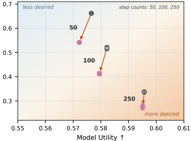
SimNPO
