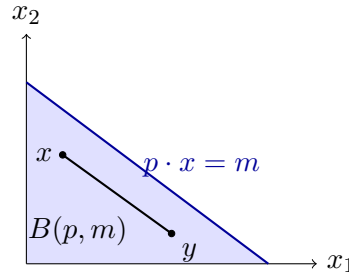
Figura 2.2: El conjunto presupuestario con dos bienes: un triángulo, que es la intersección de tres semiespacios ( x_1 \geq 0 , x_2 \geq 0 , p \cdot x \leq m ). El segmento entre dos canastas asequibles queda dentro del conjunto.
