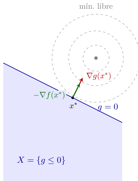
Figura 9.1: Una restricción activa: en el óptimo x^* , la curva de nivel de f (líneas discontinuas) es tangente a la frontera \{g = 0\} y -\nabla f(x^*) es un múltiplo no negativo de \nabla g(x^*) . El mínimo sin restricciones queda fuera de la región factible.
