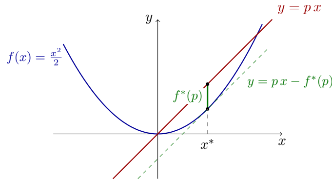
Figura 12.1: La conjugada f^*(p) es la brecha vertical máxima entre la recta y = px y la gráfica de f ; se alcanza en el punto x^* donde la pendiente de f iguala a p . Al bajar la recta y = px exactamente f^*(p) unidades se obtiene la recta soporte de pendiente p (línea discontinua).
