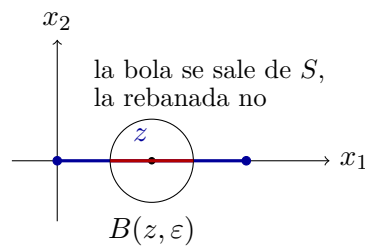
Figura 2.3: El segmento S \subseteq \mathbb{R}^2 tiene interior vacío: ninguna bola bidimensional cabe en él. Pero la intersección de la bola con \text{aff } S (el trazo grueso sobre el eje) sí cabe: z \in \text{ri } S .
