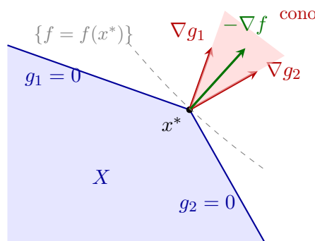
Figura 9.2: Dos restricciones activas (solución de esquina): la optimalidad exige que -\nabla f(x^*) esté en el cono generado por \nabla g_1(x^*) y \nabla g_2(x^*) (región sombreada). Ya no hay tangencia con ninguna frontera individual.
