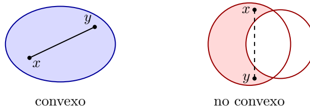
Figura 2.1: A la izquierda, un conjunto convexo: el segmento entre dos puntos cualesquiera queda dentro. A la derecha, un conjunto con forma de luna: el segmento punteado entre x e y sale del conjunto.
