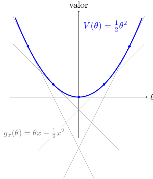
Figura 11.1: La función de valor V(\theta) = \frac{1}{2}\theta^2 (curva gruesa) como envolvente superior de la familia de rectas g_x(\theta) = \theta x - \frac{1}{2}x^2 (una recta por cada decisión congelada x \in \{-2, -1, 0, 1, 2\} ). Cada recta queda debajo de V y la toca tangencialmente en \theta = x , donde esa decisión es la óptima.
