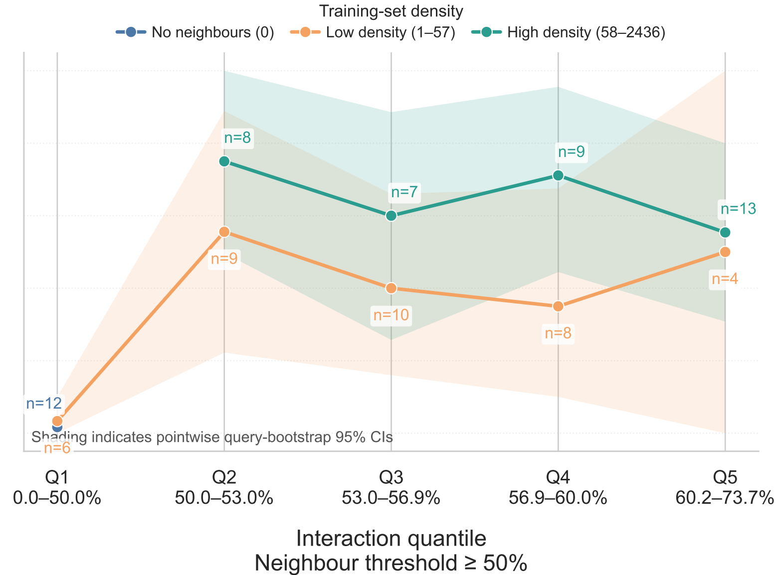
Boltz-2
