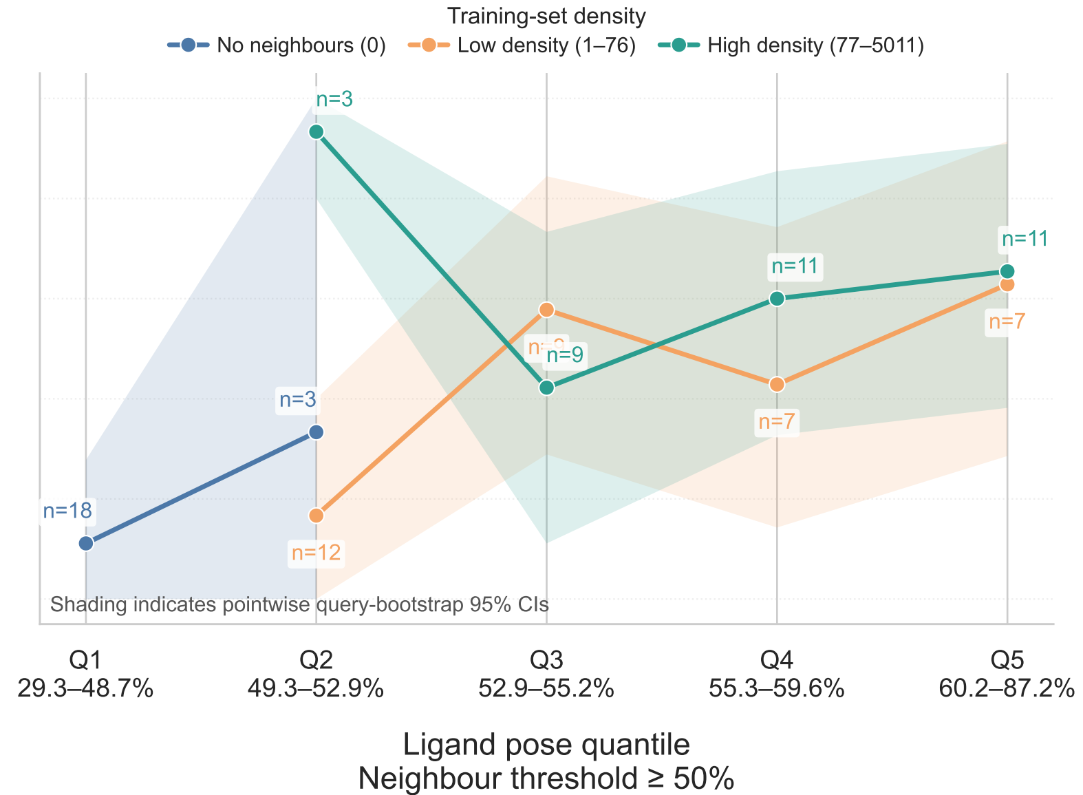
Boltz-2
