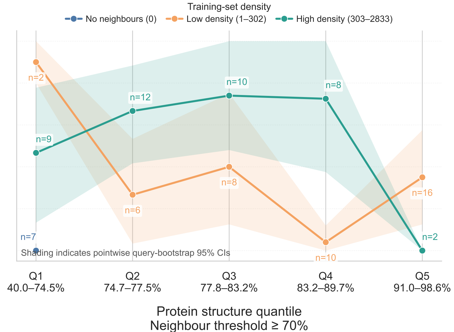
Boltz-2
