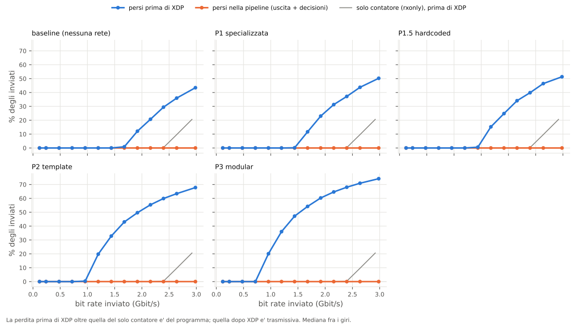
Perdita contro bit rate inviato — frame 64 B
