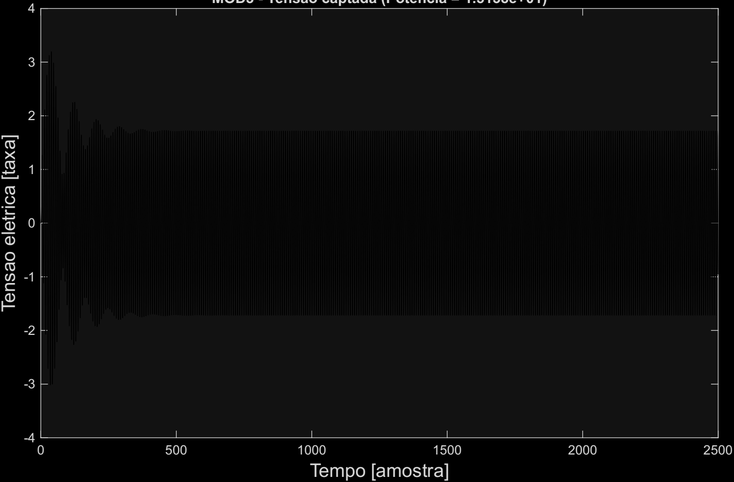
MOD3 - Tensao captada (Potencia = 1.5138e+01)
