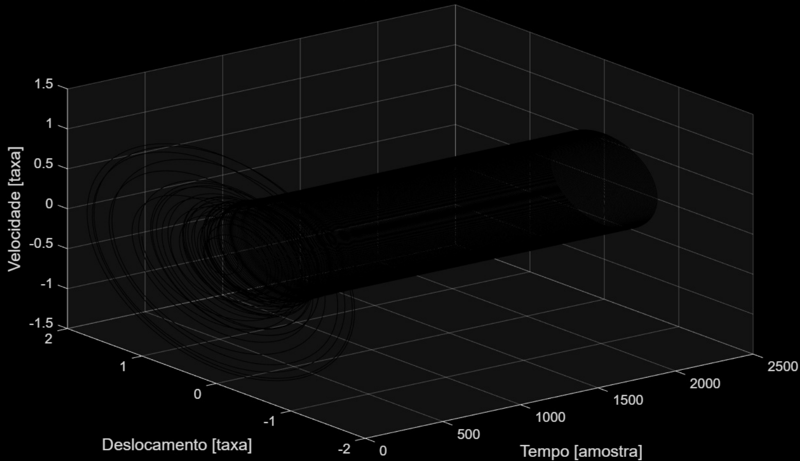
BASE - Retrato de fase 3D
