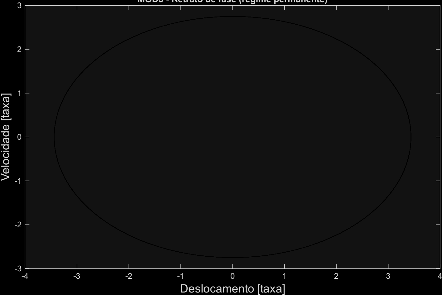
MOD3 - Retrato de fase (regime permanente)
