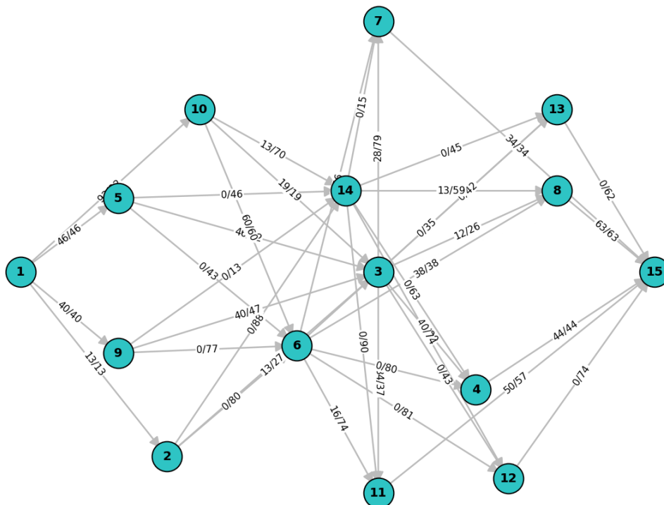
Figura 11: Fluxo ótimo (rótulos fluxo/capacidade ) — Ex. 5.
