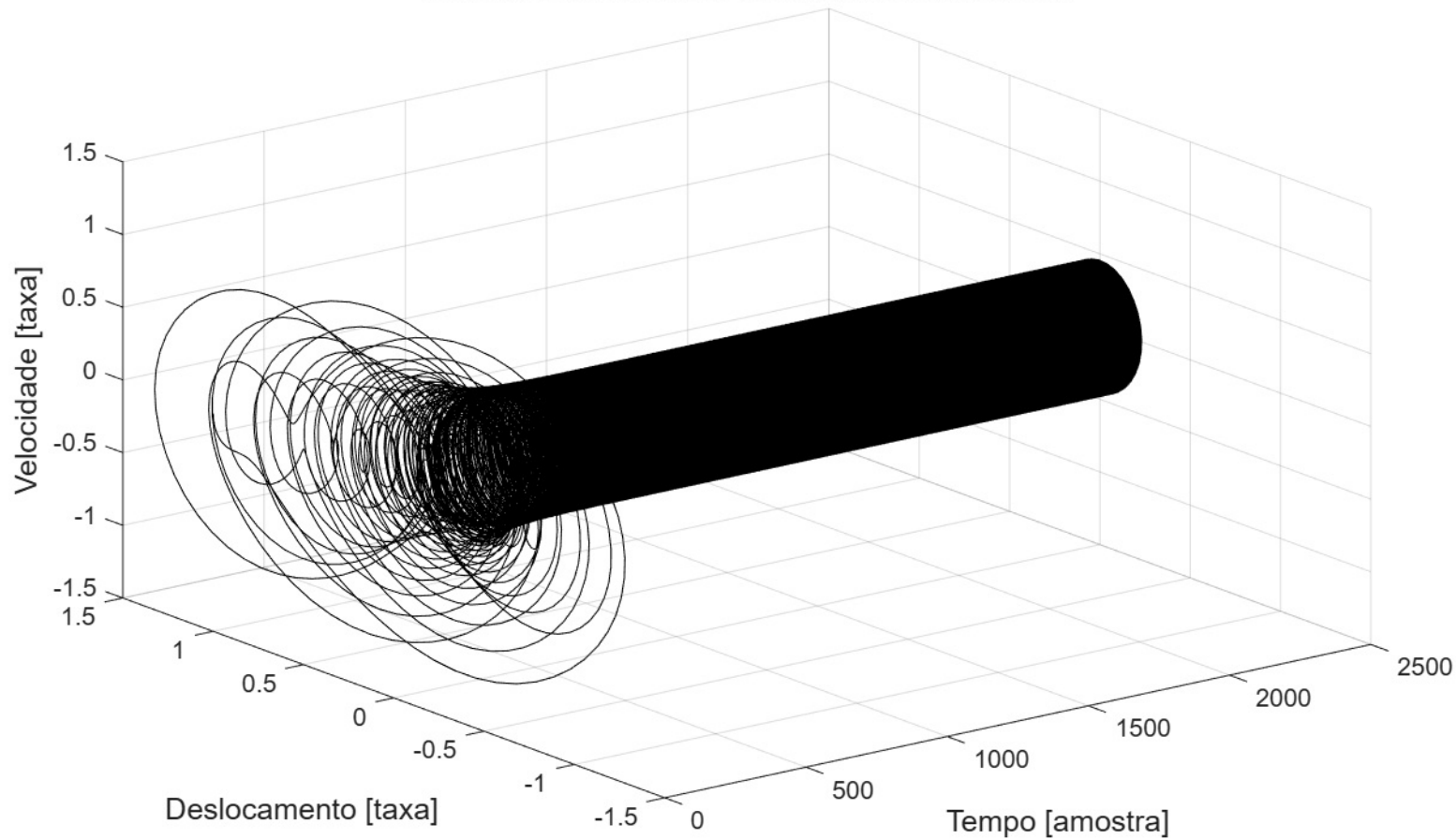
Sistema 1: Linear com Excitacao Nao-Ideal - MOD
