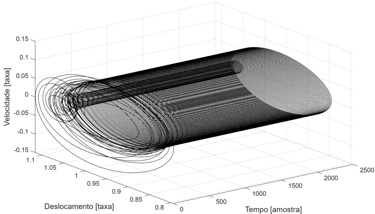
Sistema 3: Nao-Linear com Excitacao Periodica - MOD
