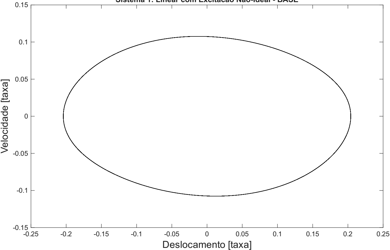
Sistema 1: Linear com Excitacao Nao-Ideal - BASE
