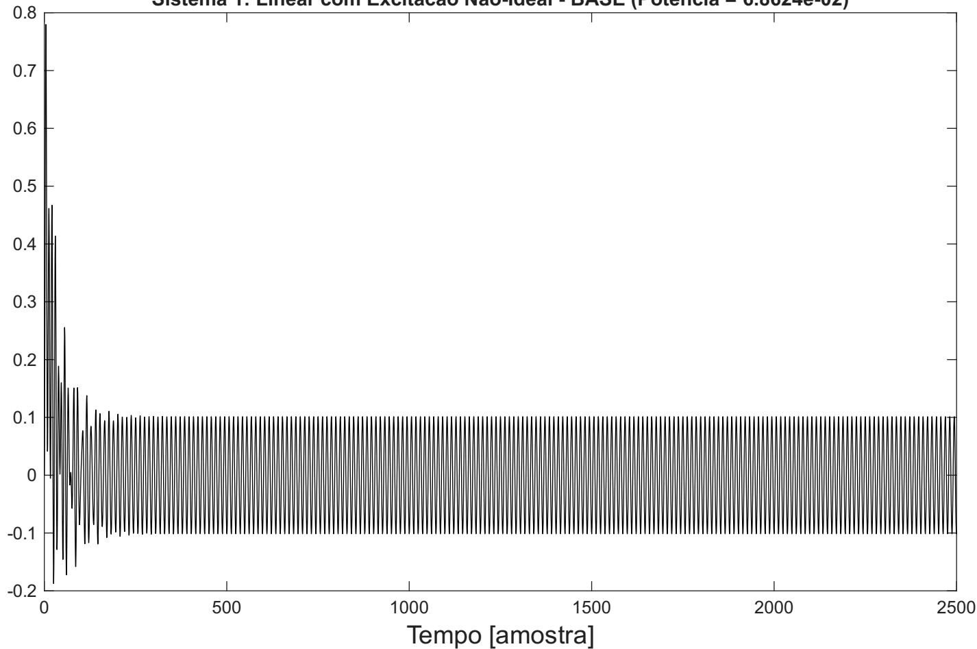
Sistema 1: Linear com Excitacao Nao-Ideal - BASE (Potencia = 6.8624e-02)
