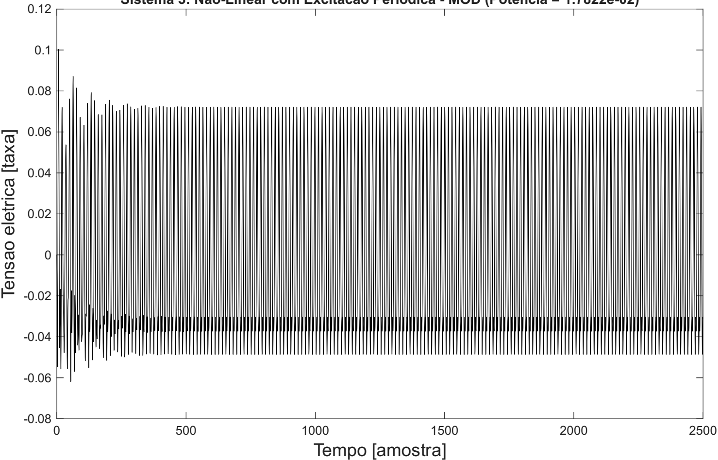
Sistema 3: Nao-Linear com Excitacao Periodica - MOD (Potencia = 1.7822e-02)
