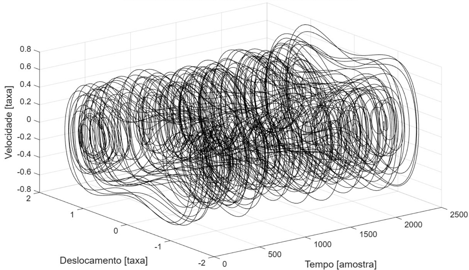
Sistema 3: Nao-Linear com Excitacao Periodica - BASE
