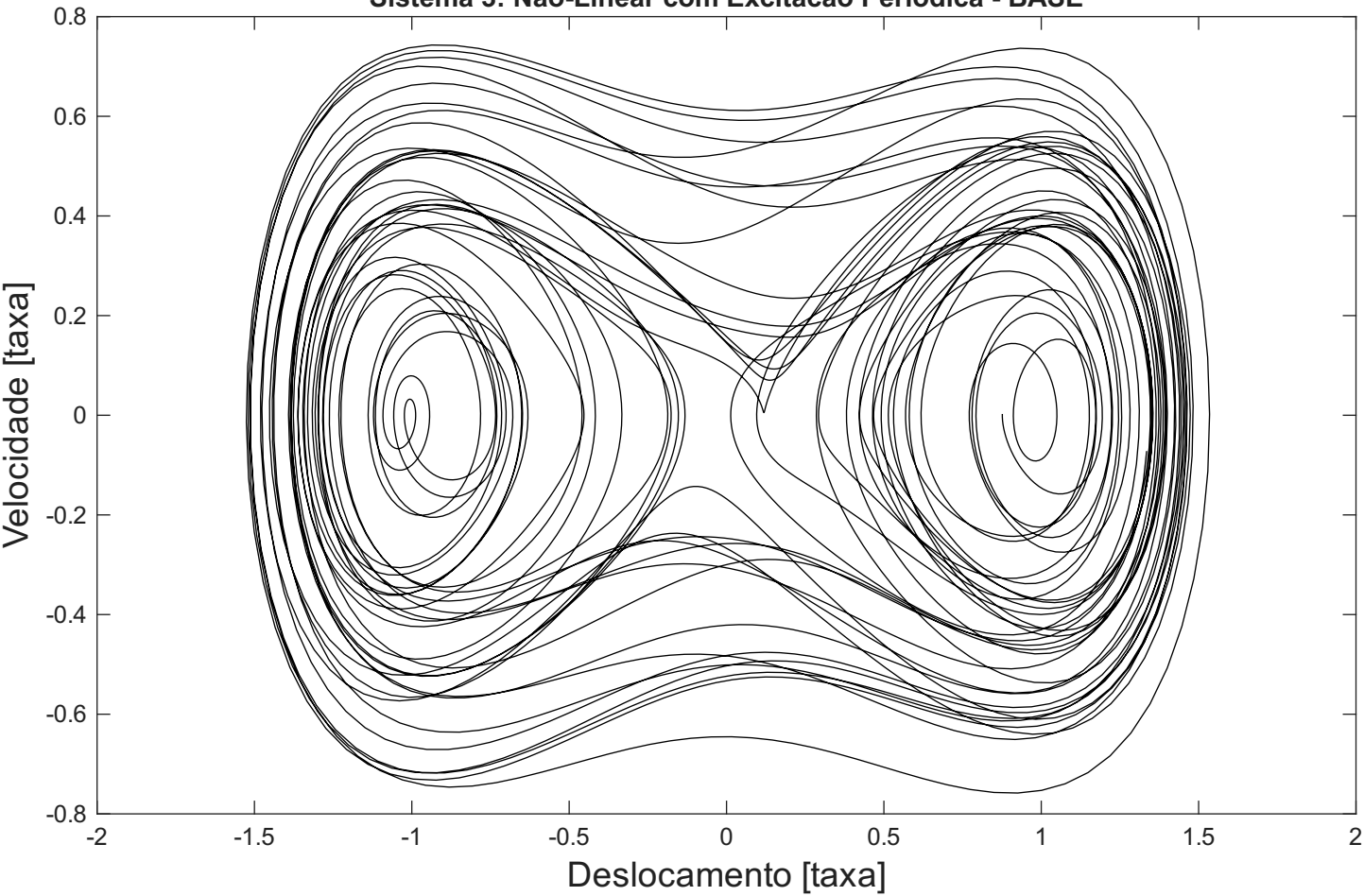
Sistema 3: Nao-Linear com Excitacao Periodica - BASE
