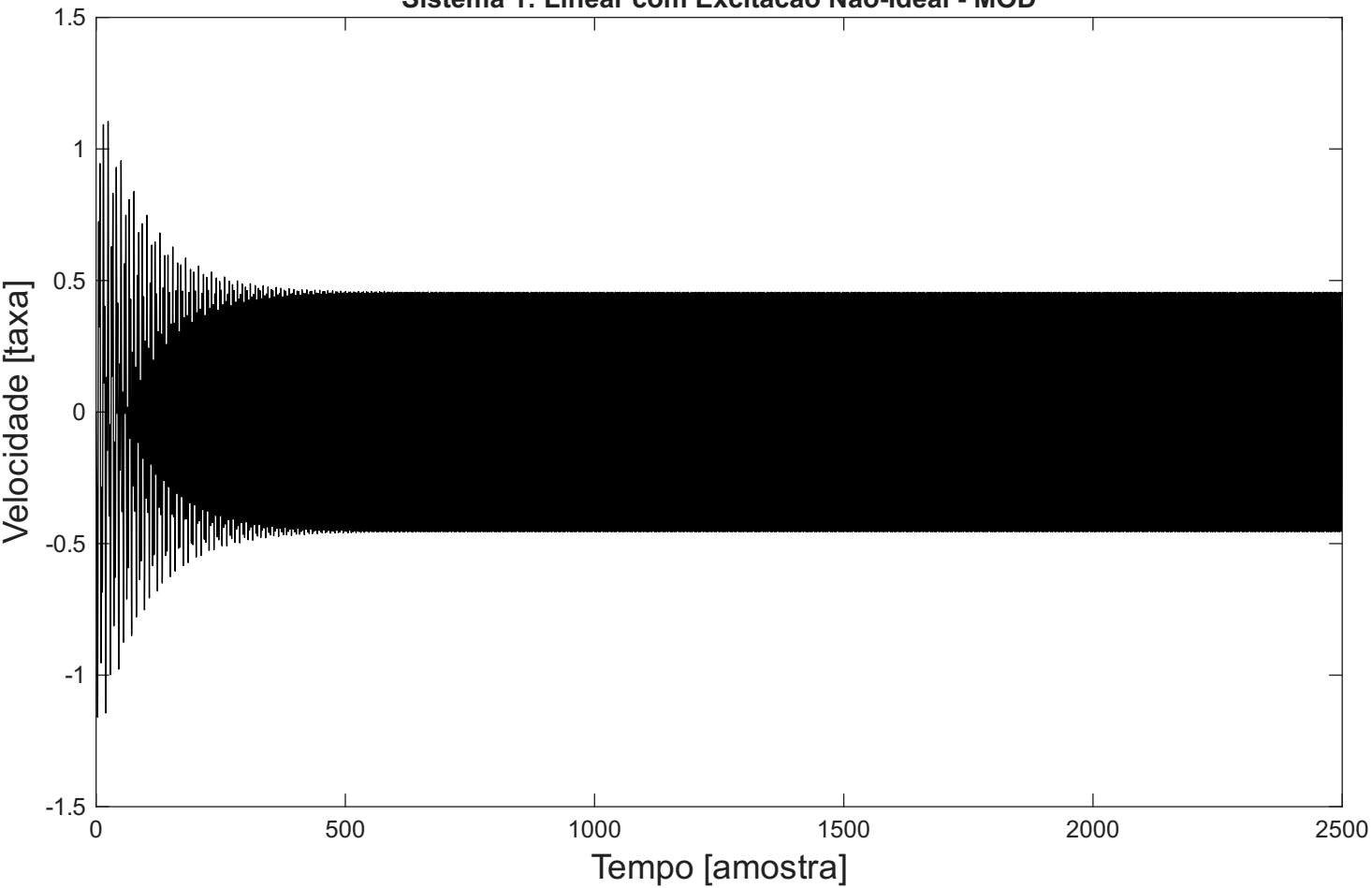
Sistema 1: Linear com Excitacao Nao-Ideal - MOD
