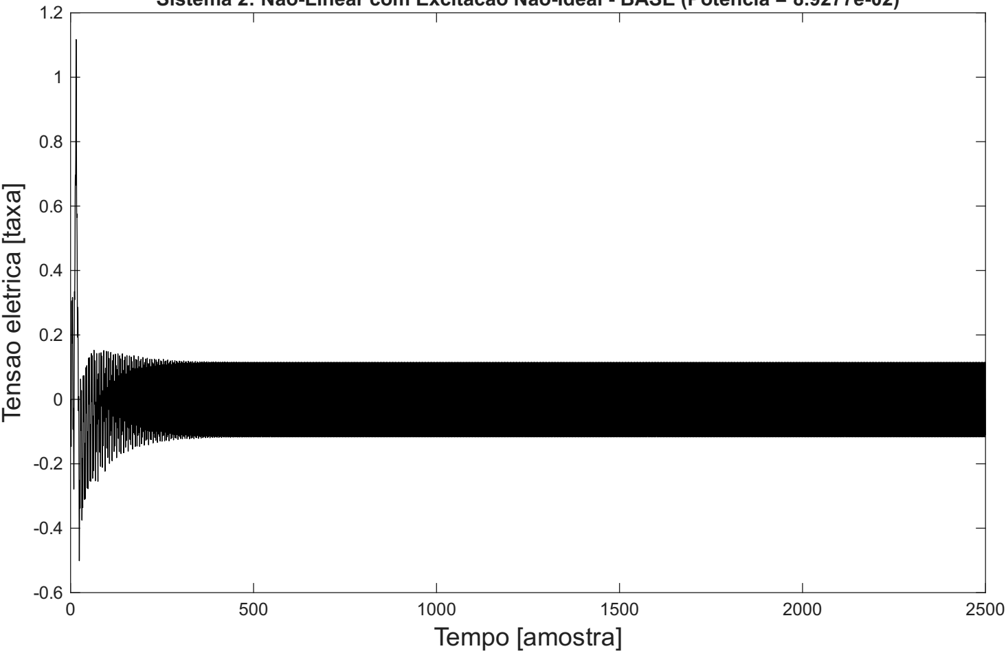
Sistema 2: Nao-Linear com Excitacao Nao-Ideal - BASE (Potencia = 8.9277\text{e-}02 )
