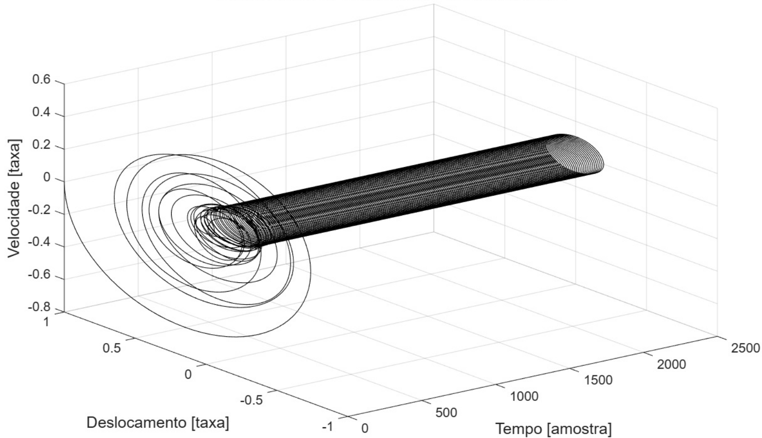
Sistema 1: Linear com Excitacao Nao-Ideal - BASE
