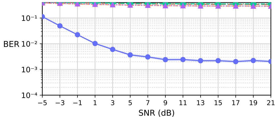
Ultra-CAN (Conv1D)
