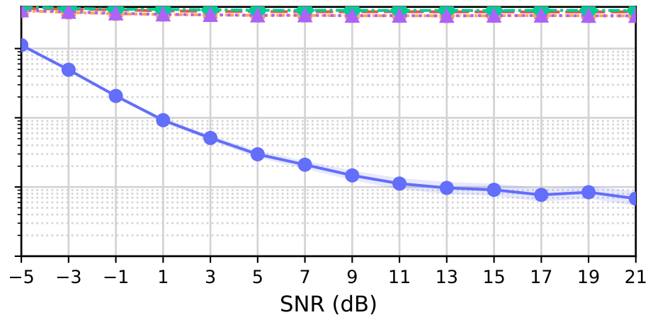
Ultra-CAN-QKV
