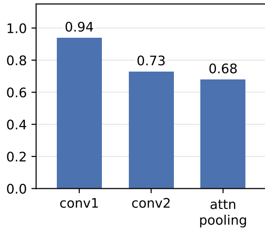
Ultra-CAN (Conv1D)
