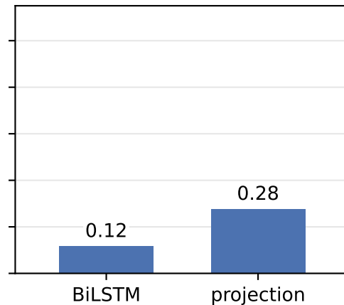
MC-DLCSK
