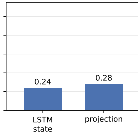
LSTM-OFDM-DCSK
