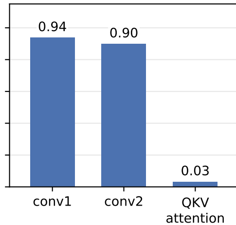
Ultra-CAN (QKV)
