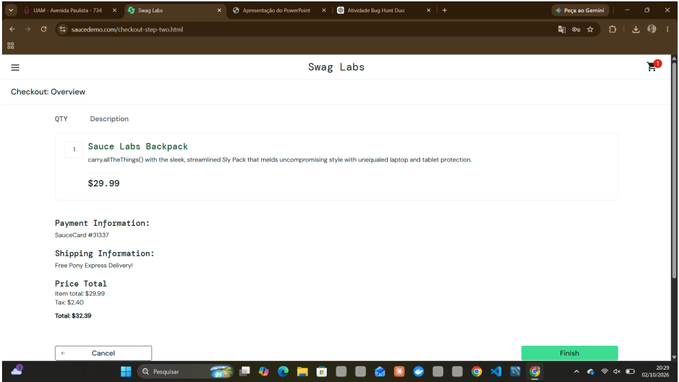
Figura 2 – Tela seguinte (checkout-step-two.html): o checkout avançou normalmente com o CEP inválido.
