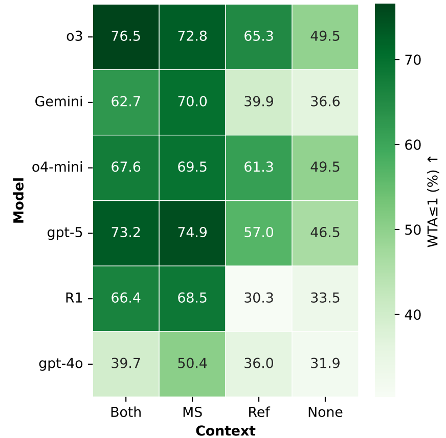
WTA ≤1 (%) ↑
