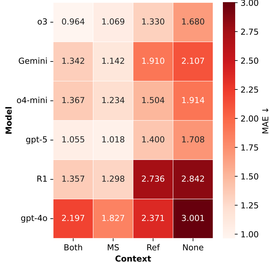
MAE ↓
