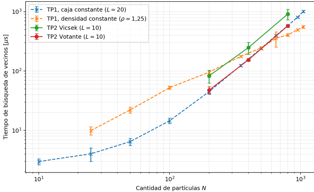
Figura 13: Tiempo de búsqueda de vecinos en función de N , en escala doblemente logarítmica. Se comparan las corridas dedicadas de este trabajo con las mediciones periódicas del TP1. Las configuraciones no son equivalentes: difieren en densidad, en L y en el número de celdas por lado.
