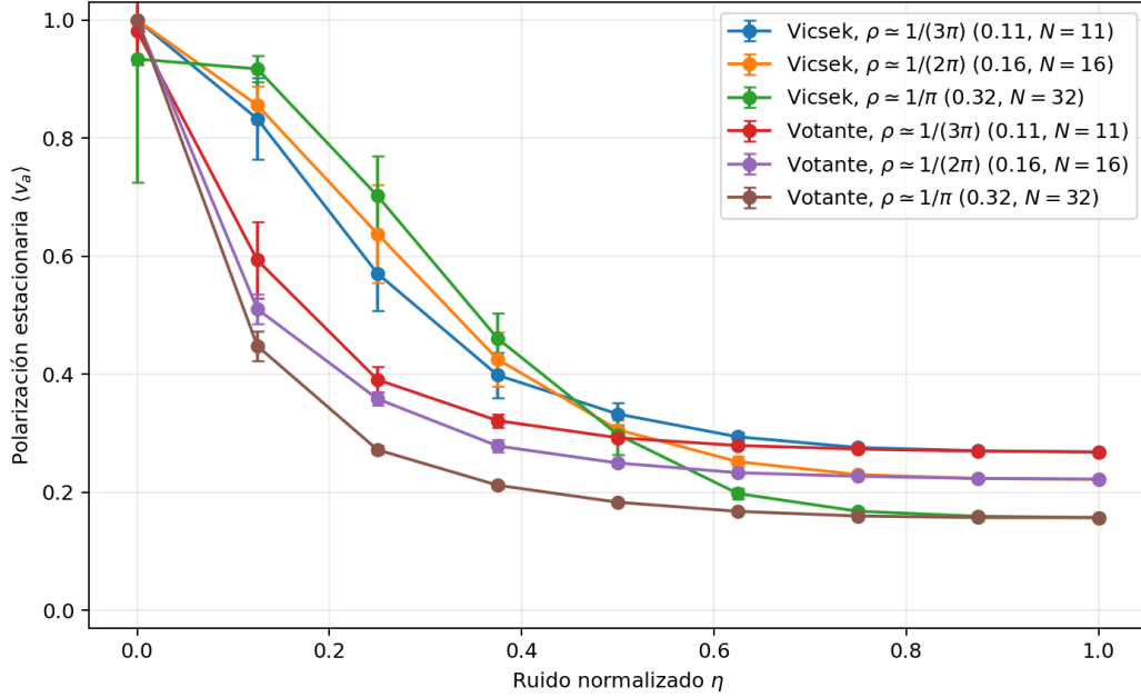
Figura 11: Polarización estacionaria en función del ruido en las densidades bajas. El valor al que satura cada curva en \eta = 1 corresponde al piso de desorden de la Ec. (10) y crece al disminuir N .
