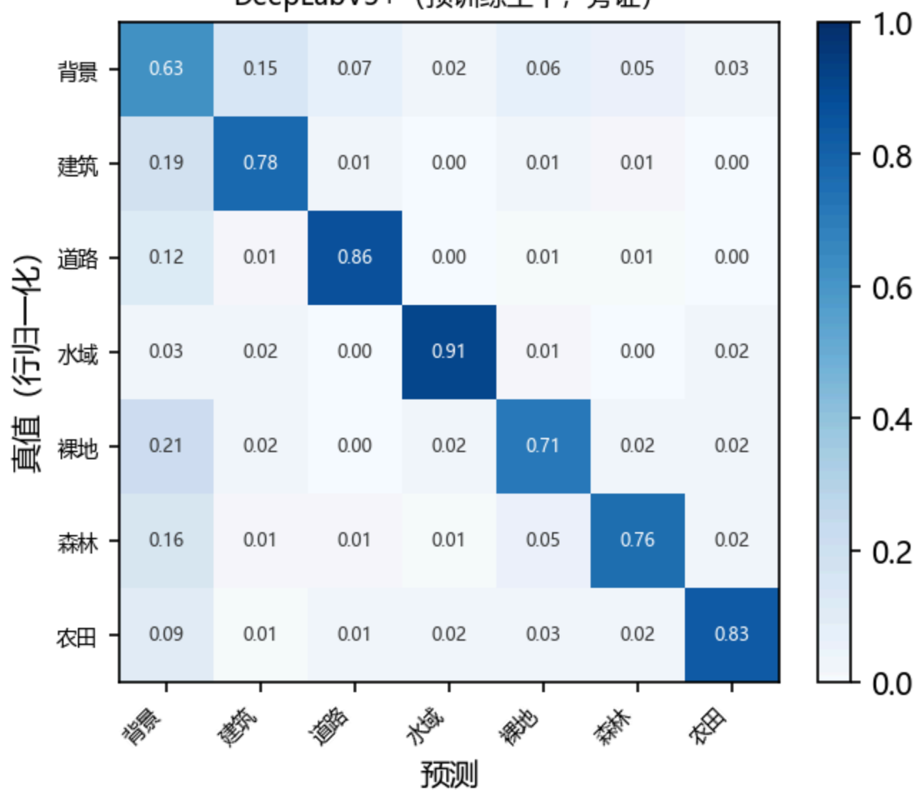
DeepLabV3+ (预训练主干, 旁证)
